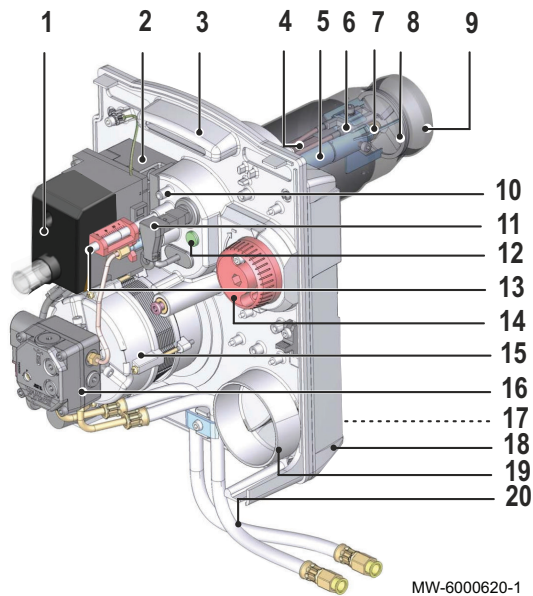
Abb.3 Hauptkomponenten
