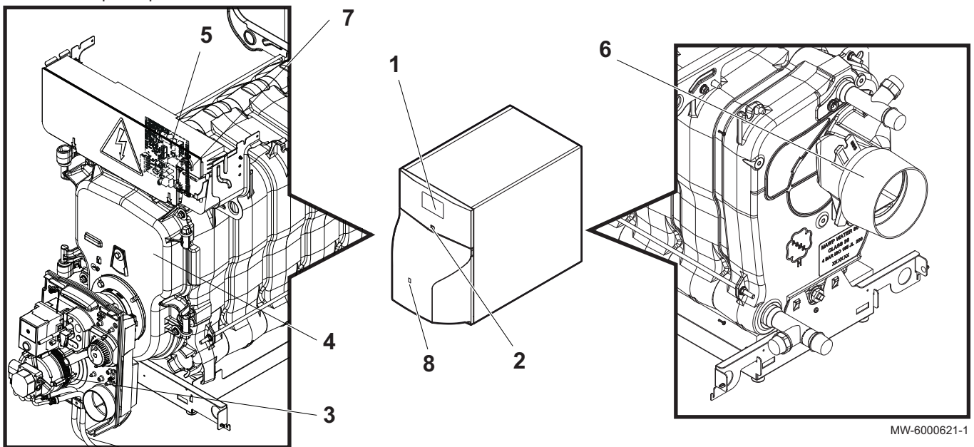
Abb.2 Hauptkomponenten
